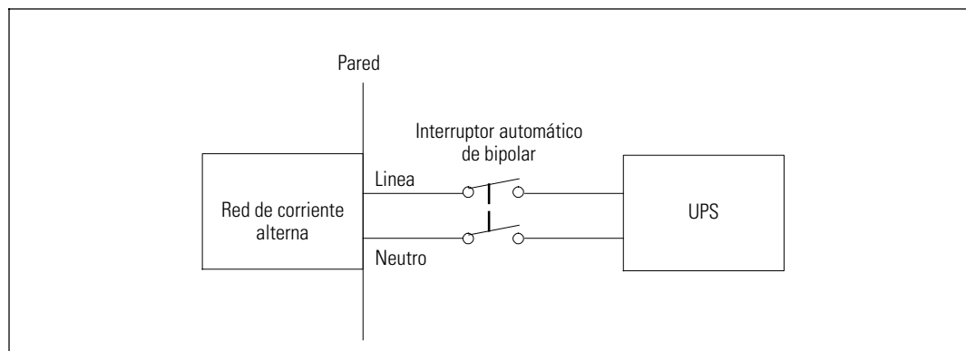
Figura 6. Disyuntor Diagrama
